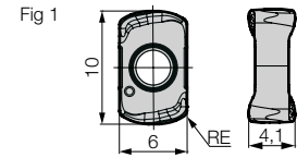
Abmessungen (mm)
