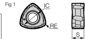
Abmessungen (mm)
